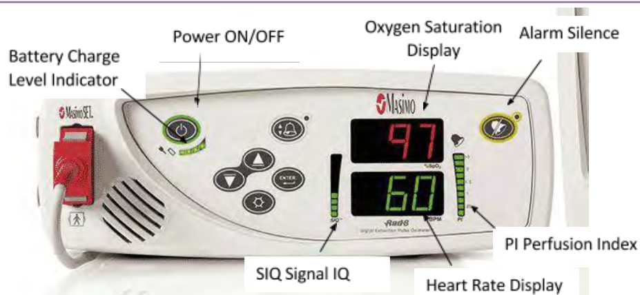
Figure 11. Masimo Rad8 Pulse Oximeter. www.dufortlavigne.com/en/produit/MAM9190
